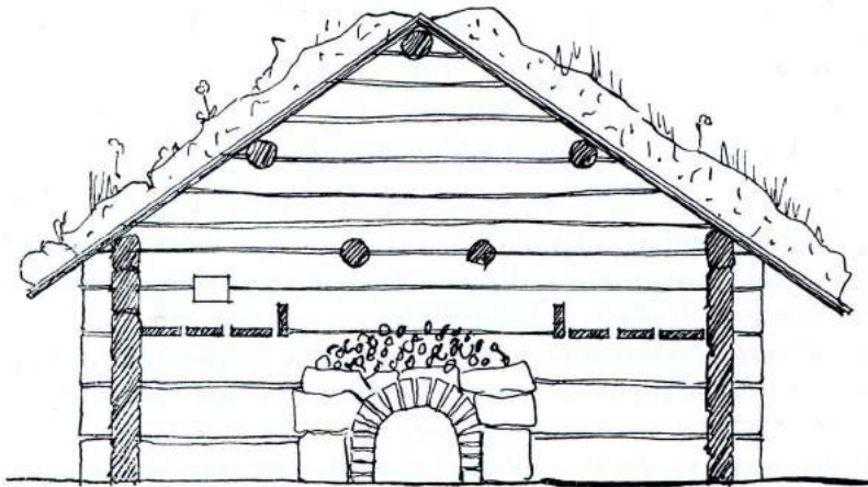
Plan och genomskärning av bastu med bastulider. Häsäng, Vattan. Nordiska museets undersökningar i Gästrikland 1920.
